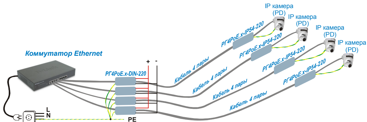
Пример использования RG4PoE.x-DIN-220 в паре с RG4PoE.x-IP54-220 на сети с применением технологии PassivePoE.
