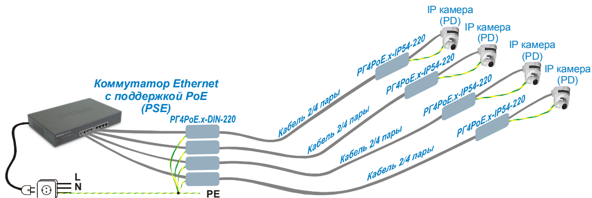
Пример использования RG4PoE.x-DIN-220 в паре с RG4PoE.x-IP54-220 на сети с применением технологии PoE (IEEE802.3af/at).
