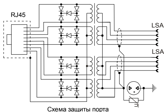
Схема защиты порта
